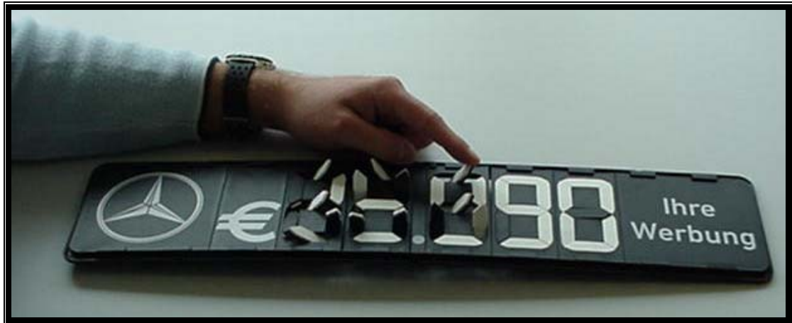
3. Bild: Der Top Pricer kann sofort verwendet werden. Der Preis wird einfach durch drehen der schwarz/weißen Balken auf einer Mittelachse individuell eingestellt!
